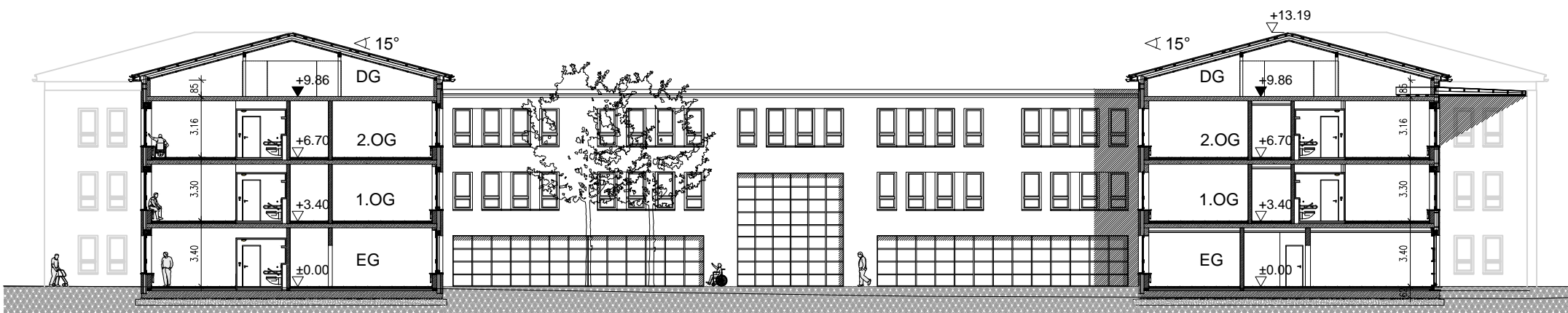
Schnitt A-A
