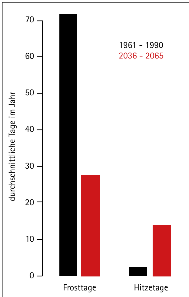
Abbildung 4: Veränderung der Frost- und Hitzetage der Station Altenburg bei Münster nach dem Szenario „RCP 8.5“, basierend auf dem STARS Modell Daten: PIK, 2013, Abbildung: Anne Holsten
