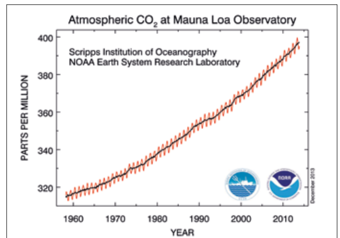
Abbildung 2: Entwicklung des CO 2 in der Atmosphäre von 1958 bis 2012, gemessen an der Station Mauna Loa, Hawaii (längste Messreihe der Welt). Die rote Kurve zeigt die monatlichen Werte. Hier erkennt man die jahreszeitlichen Schwankungen, die v.a. durch Pflanzen verursacht werden. Die schwarze Kurve zeigt die jährlichen Werte. Quelle: Dr. Pieter Tans, NOAA/ESRL ( www.esrl.noaa.gov/gmd/ccgg/trends/ ) and Dr. Ralph Keeling, Scripps, Institution of Oceanography ( scrippsco2.ucsd.edu/ ). http://www.esrl.noaa.gov/gmd/ccgg/trends/mlo.html
