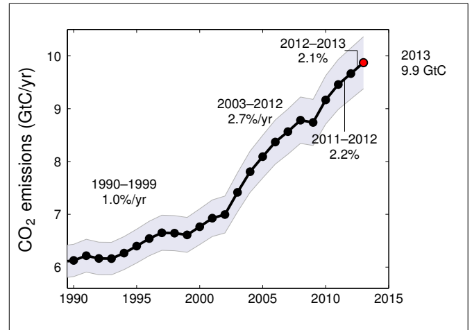
Abbildung 1: Globale CO 2 -Emissionen aus der Verbrennung von fossilen Energieträgern und der Zementproduktion. Die Prozentzahlen geben die jährliche Steigerung an, der rote Punkt stellt die Schätzung für 2013 dar. Quelle: Le Quéré et al 2013; CDIAC Data; Global Carbon Project 2013, http://www.globalcarbonproject.org
