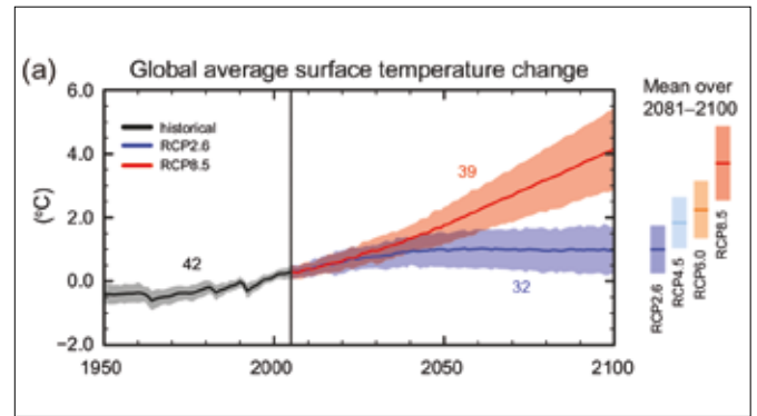
Abbildung 3: Veränderung der globalen Jahresmitteltemperatur bis 2100 im Vergleich zu den Jahren 1986-2005 auf Basis der RCP Szenarien und verschiedenen Klimamodellen, deren Anzahl jeweils innerhalb des Diagramms angegeben ist) Quelle: IPCC 2013
