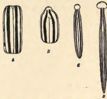
Fig. 5. Stück des Wurm Bipalium (A), das sich zu einem neuen Tier umbildet (B, C, D). (Nach Morgan).
