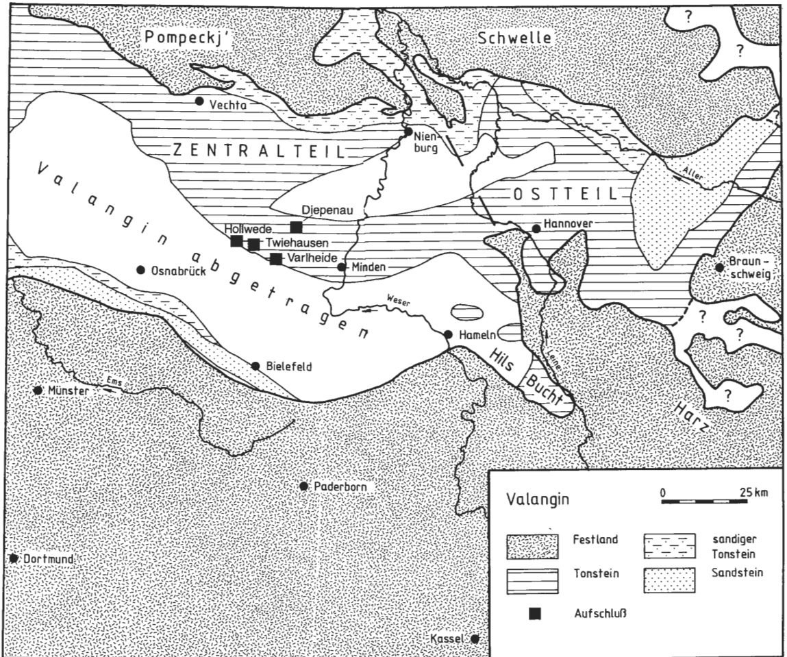
Abb. 3: Paläogeographische Karte des zentralen Teils des nw-deutschen Beckens im Valangin (geändert nach Schott et al. 1967, 1969). Die gestrichelte Gerade W Hannover stellt die Grenze zwischen Zentral- und Ostteil dar.
