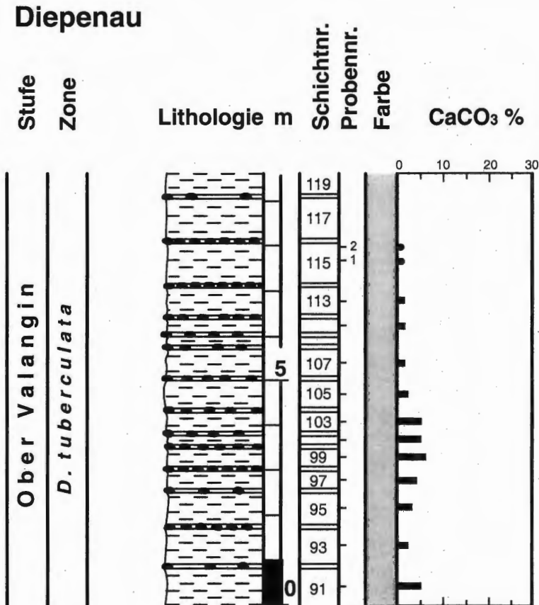
Abb. 23: Lithologie und Stratigraphie des Profils Diepenau.
