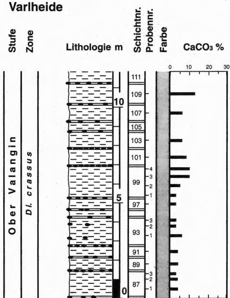
Abb. 17: Lithologie und Stratigraphie des Profils Varlheide.
