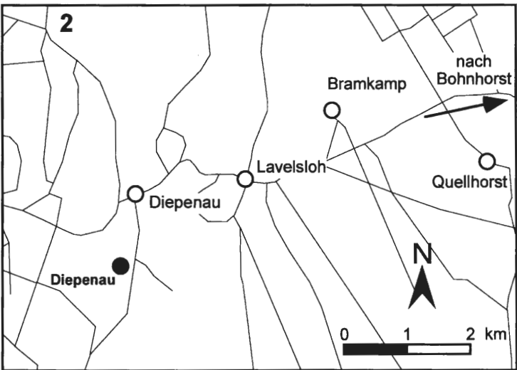
Abb. 1: Übersichtskarte des Arbeitsgebietes und Detailkarten (1, 2) mit Lage der beschriebenen Aufschlüsse Twiehausen, Hollwede, Varlheide und Diepenau.
