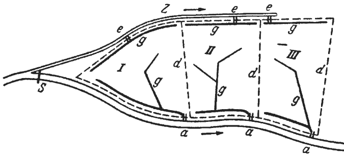
Abb. 12: Schematische Darstellung einer einfachen Überstauungsanlage (aus SCHROEDER 1958). I-III = Abteilungen, d = Dämme, Z = Zuleiter, S = Stauschleuse, e = Einlassschleusen, a = Auslassschleusen, g = Entwässerungsgräben.
