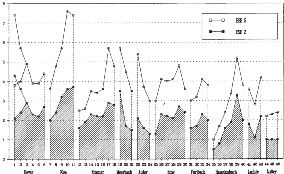
Abb. 13: Durchschnittliche Werte von BSB 2 und BSB 5 an den Probepunkten
