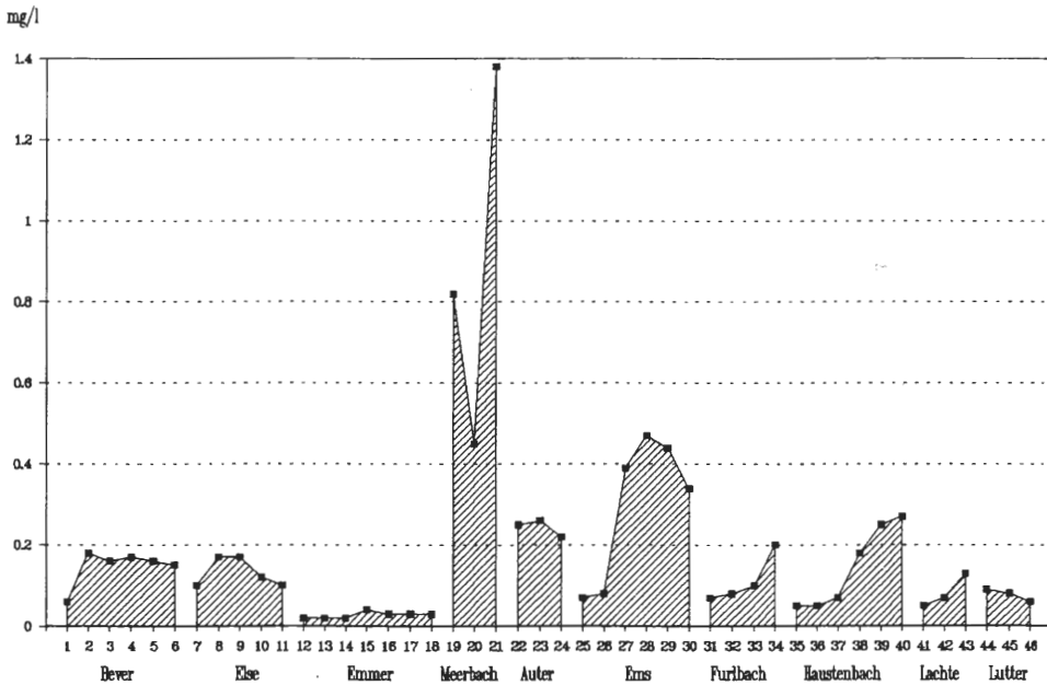
Abb. 20: Durchschnittliche Konzentrationen des Eisen-II an den Probenpunkten
