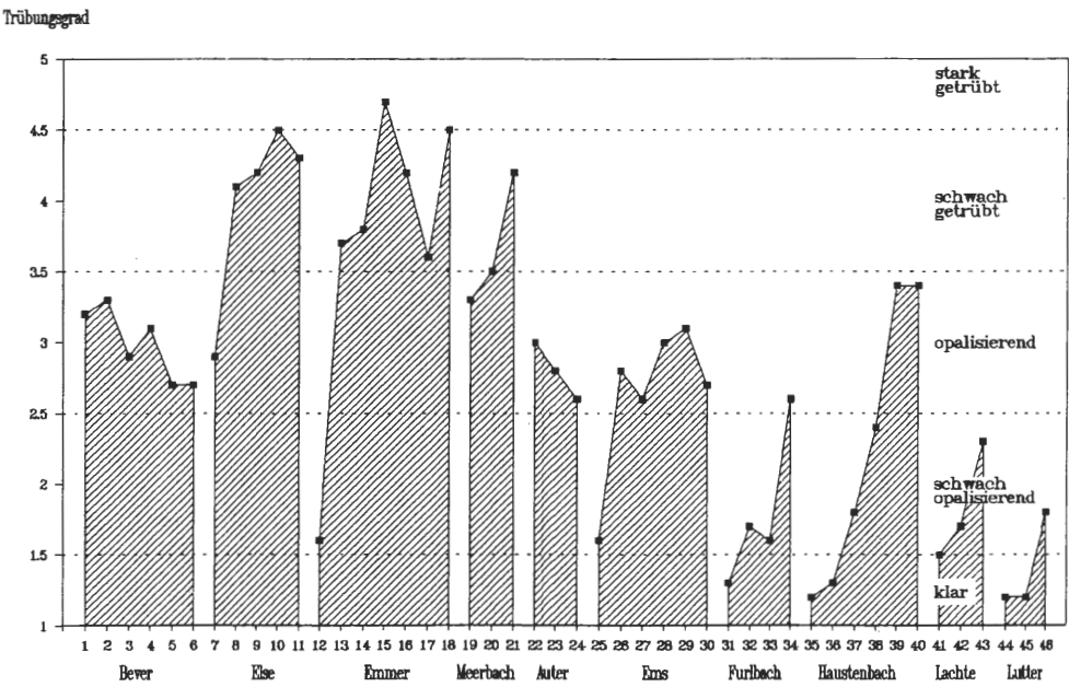
Abb. 23: Durchschnittlicher Trübungsgrad an den Probepunkten
