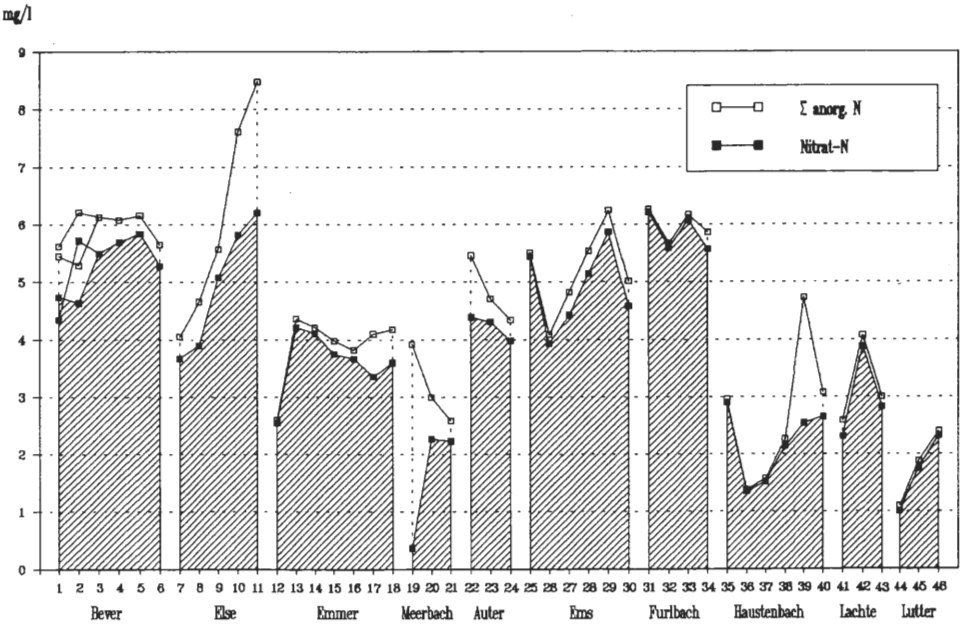
Abb. 14: Durchschnittliche Konzentrationen des Nitrat-N und der Summe anorganischen Stickstoffs an den Probepunkten
