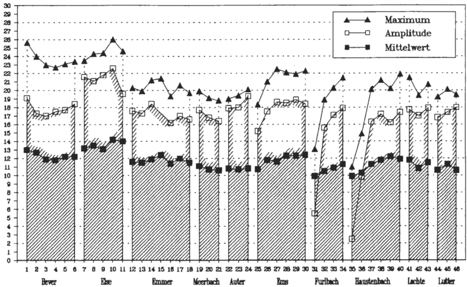
Abb. 21: Mittel- und Maximalwerte sowie Amplitude der Wassertemperatur an den Probepunkten
