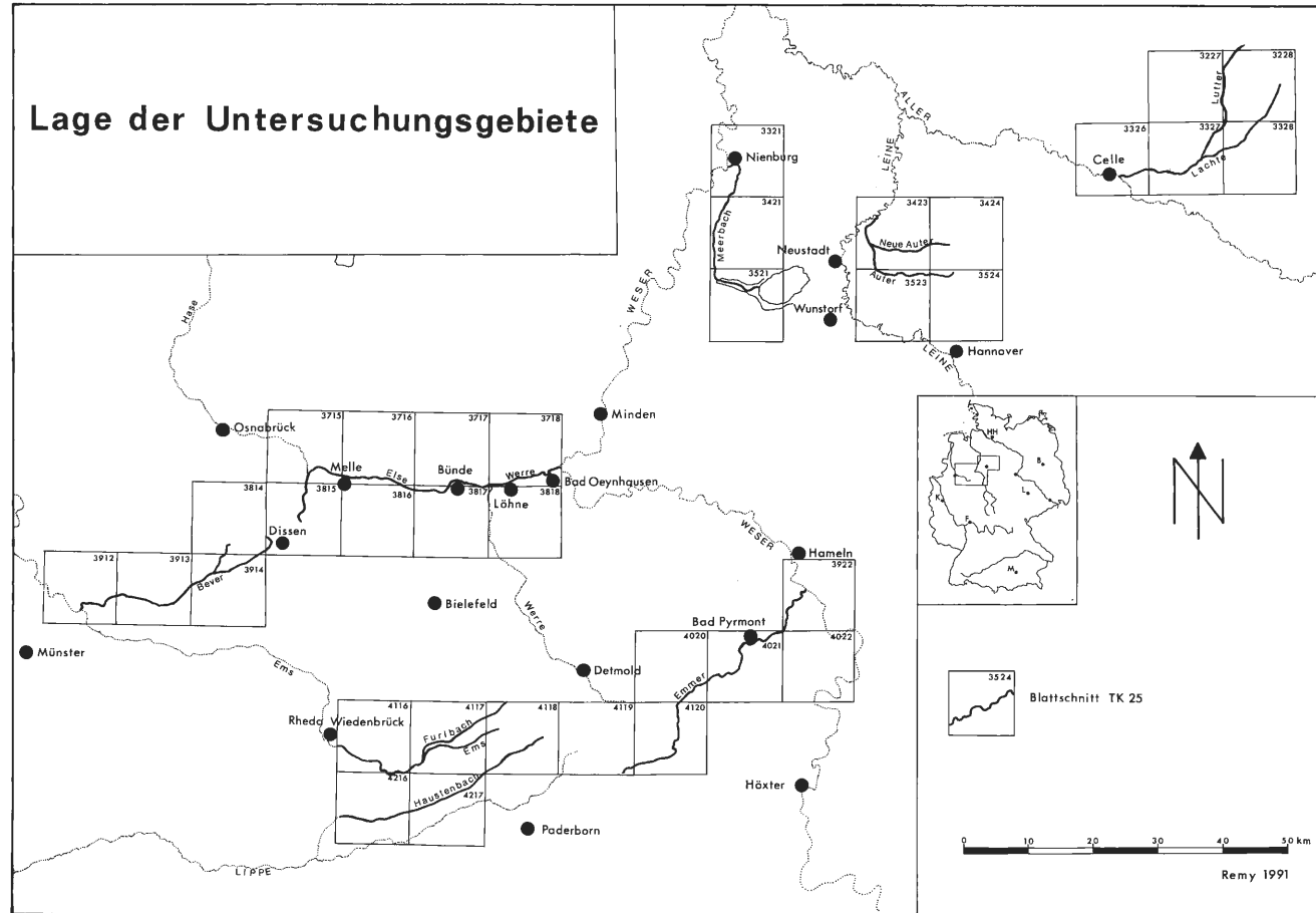
Abb. 1: Lage der untersuchten Fließgewässer mit Angabe der zugrundeliegenden TK 25 Blattschnitte
