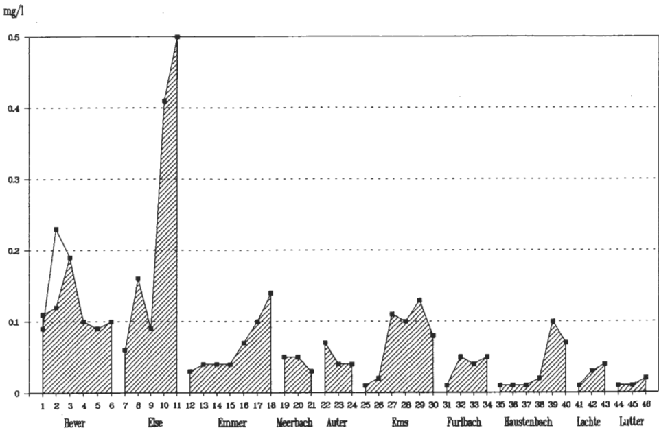
Abb. 15: Durchschnittliche Konzentrationen des Nitrit-N an den Probepunkten
