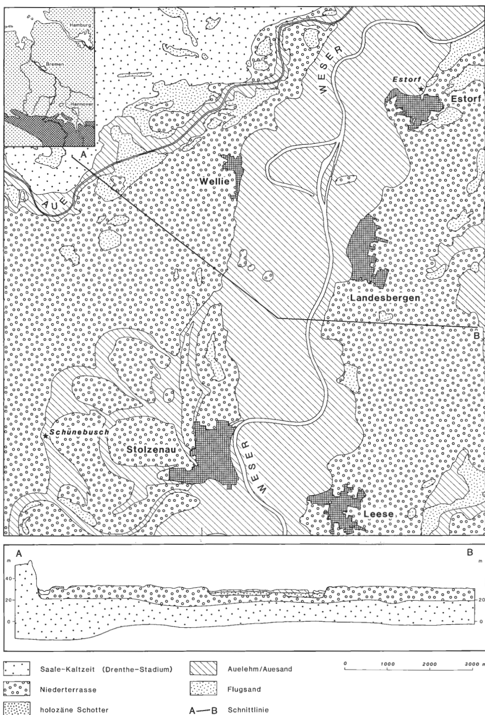
Abb. 1: Geologische Übersichtskarte und Lage des Untersuchungsgebietes (verändert nach: Geolog. Karte von Niedersachsen 1:25000; Blatt 3320 Liebenau, LÜTTIG & MEYER 1980, und 3420 Stolzenau, HÖFLE 1981)
