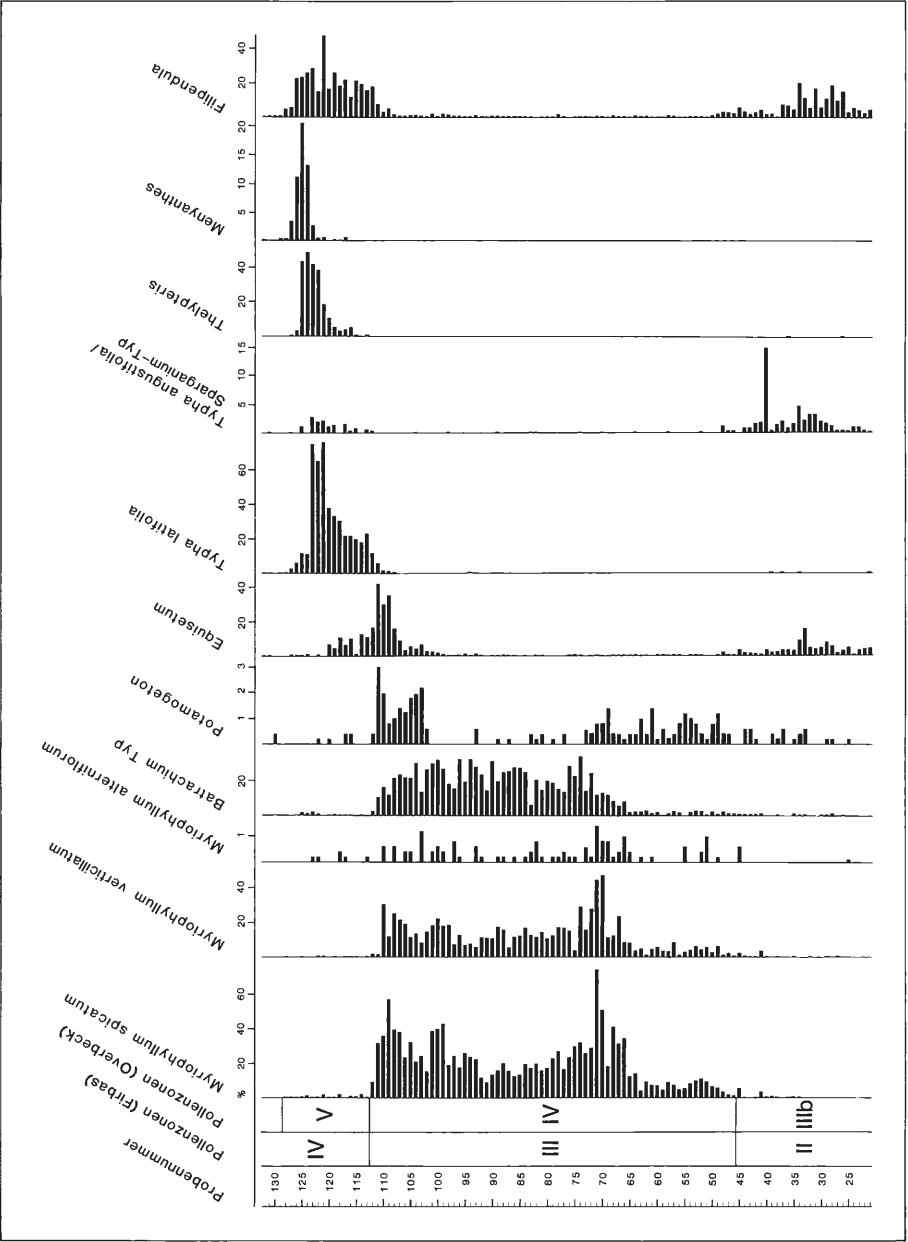
Abb. 36: Verlandungssukzession des Paläomäanders am Schönebusch
