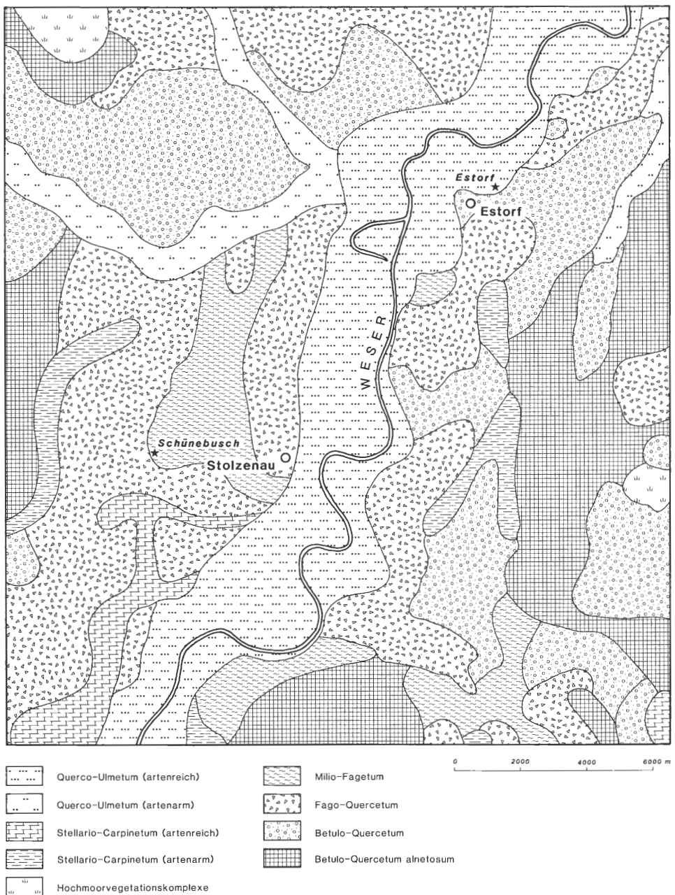
Abb. 3: Übersichtskarte der potentiellen natürlichen Vegetation (verändert nach: BURRICHTER, POTT & FURCH 1988)
