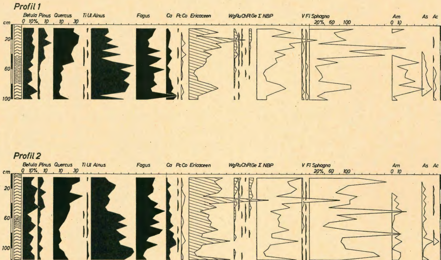
Abb. 8. Vinter Moor, Profile 1 und 2.
