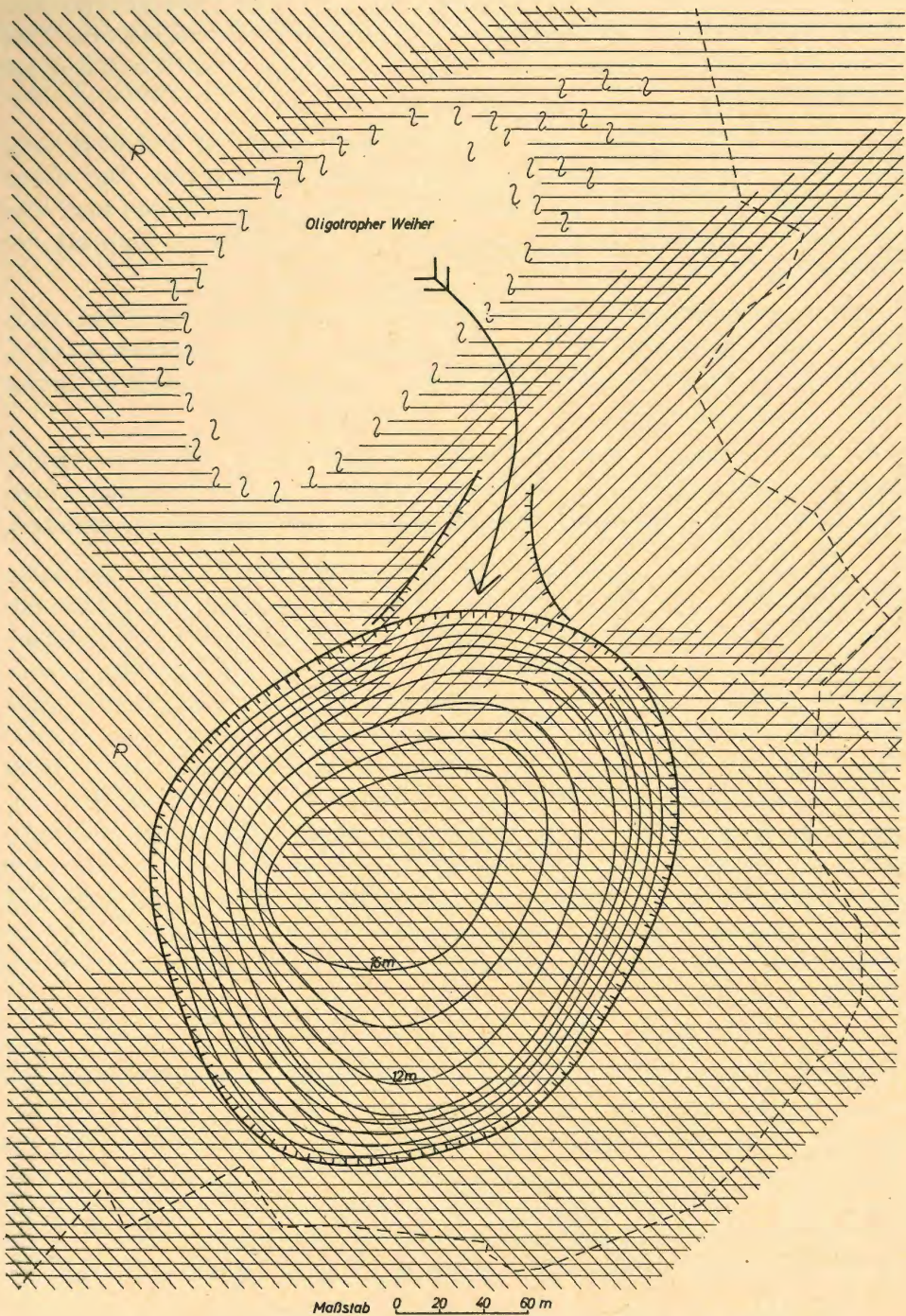
Abb. 9. Vermutliche Vegetation vor dem Einbruch und Gestalt des Einbruchskessels Zeichenerklärung siehe bei Abb. 11.
