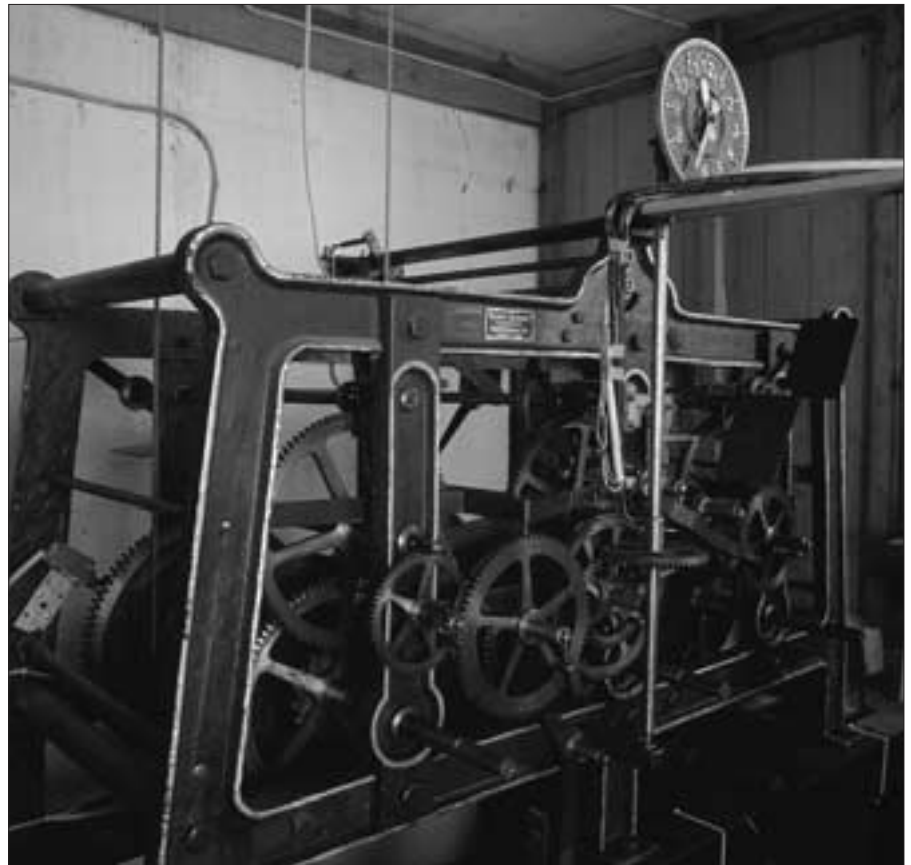
Die Turmuhr der Firma Vortmann, Recklinghausen (1947)
