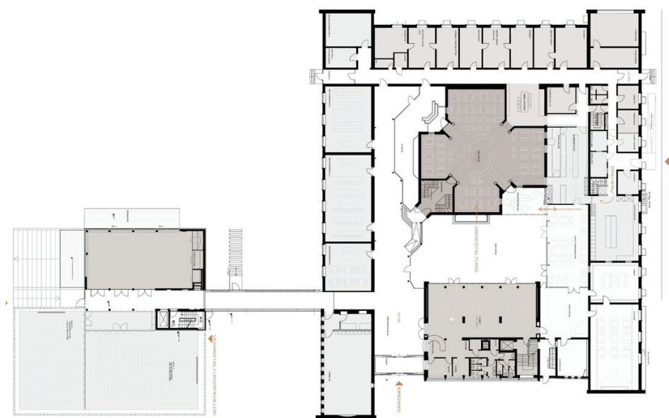
Ort: Kardinal-von-Galen-Ring 50, Münster Bauherr: Bischöfliches Generalkurienamt, Münster Architekt: kresings GmbH, Münster [LP 1-9] Volumen: 756qm BGF Fertigstellung: 2012
