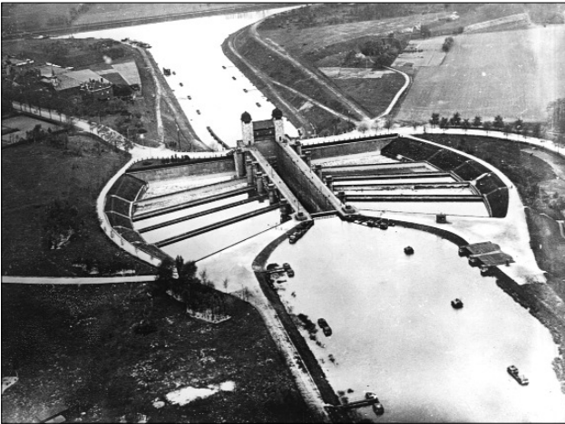
Schiffshebewerk Henrichenburg in Waltrop, Recklinghausen, ca. 1930 Fotograf unbekannt
